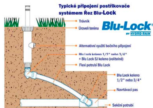
Typické připojení postřikovače systémem Řez Blu-Lock Blu-Lock® HYDRO-RAIN Systém připojení postřikovačů Blu Lock® strana 23
