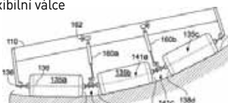
Flexibilní válce
